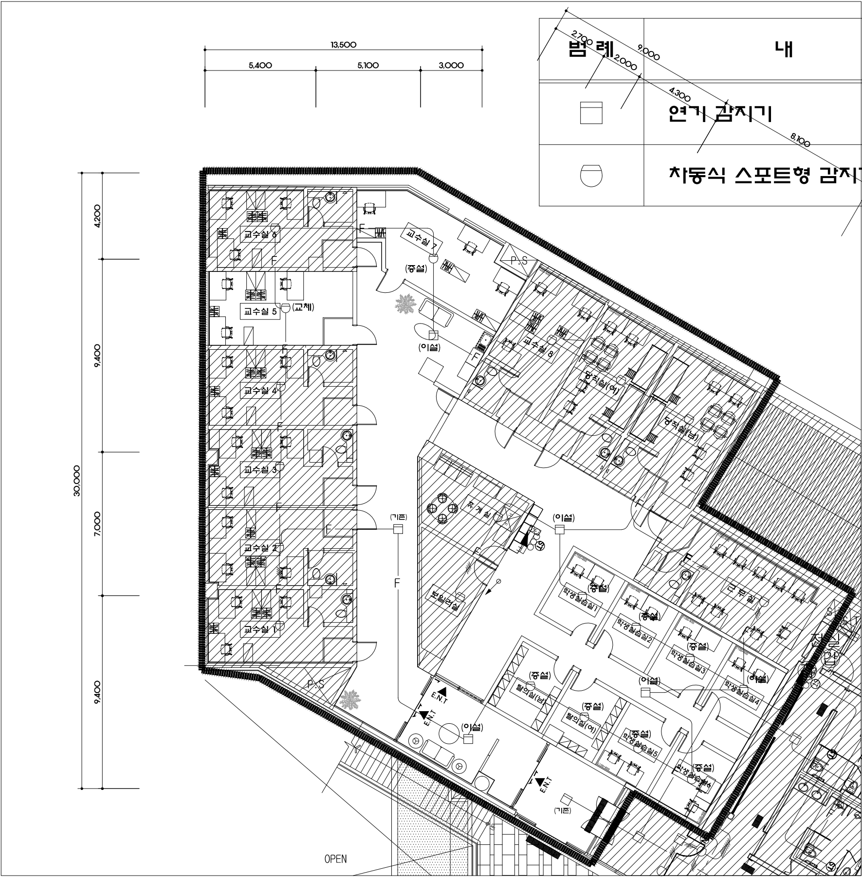
5연구실(수련시설) 자동화재탐지설비 확대평면도(변경전)
