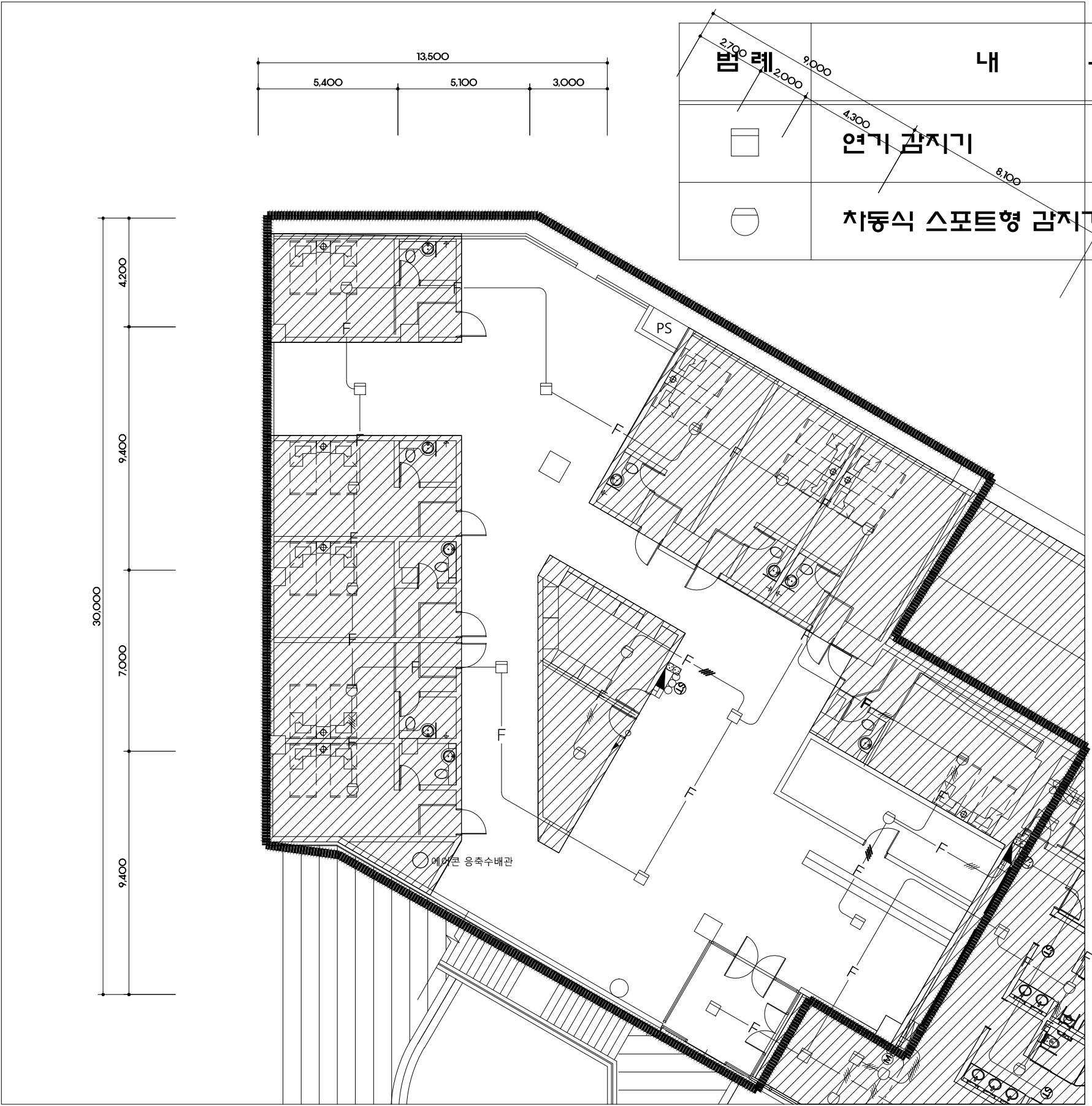
5연구실(수련시설) 자동화재탐지설비 확대평면도(변경전)
