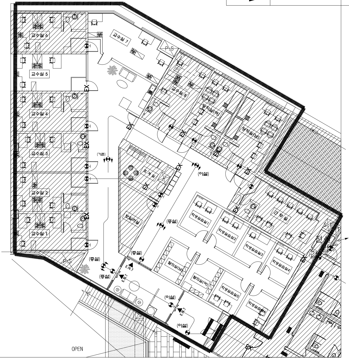
5연구실(수련시설) 유도등설비 확대평면도(변경 후)
