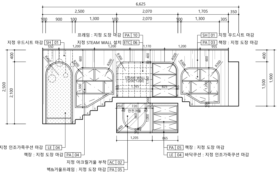
01 ELEVATION-A
